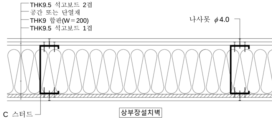
그림 3 — 스테드
