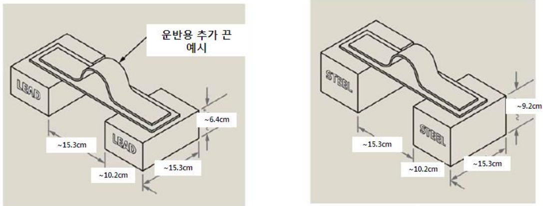
그림 E.1 — 시험추의 제작 방법 보기
