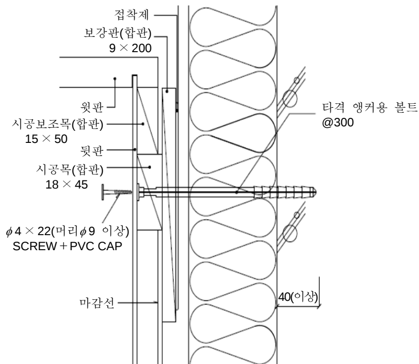
그림 6 — 단열재가 적용된 벽체
