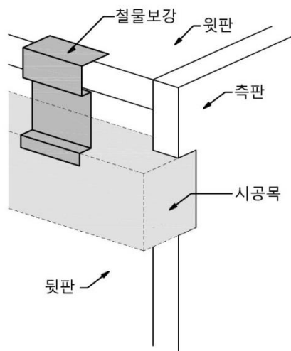
그림 D.5 — 철물보강물의 보기
