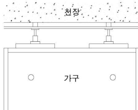
그림 12 — 전도 방지물 및 적용 위치
