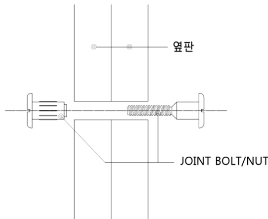
그림 C.1 — 가구와 가구 고정철물
