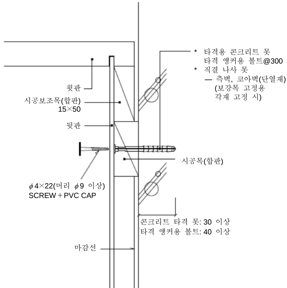
그림 1 — 시공목 고정
