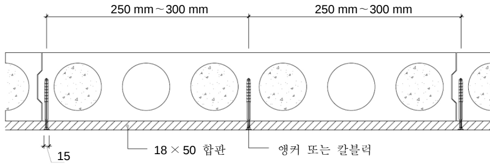
그림 5 — 압출성형 경량콘크리트 패널
