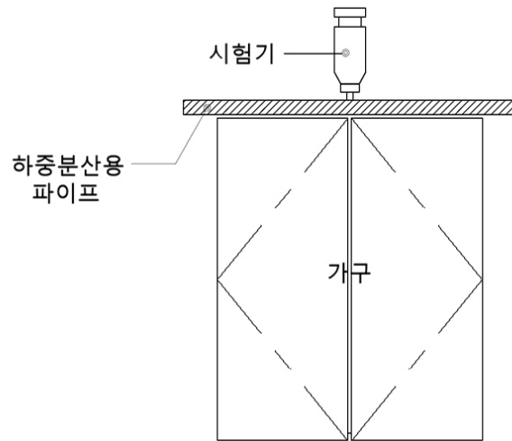
그림 A.1 — 시험기를 가구에 설치하는 방법
