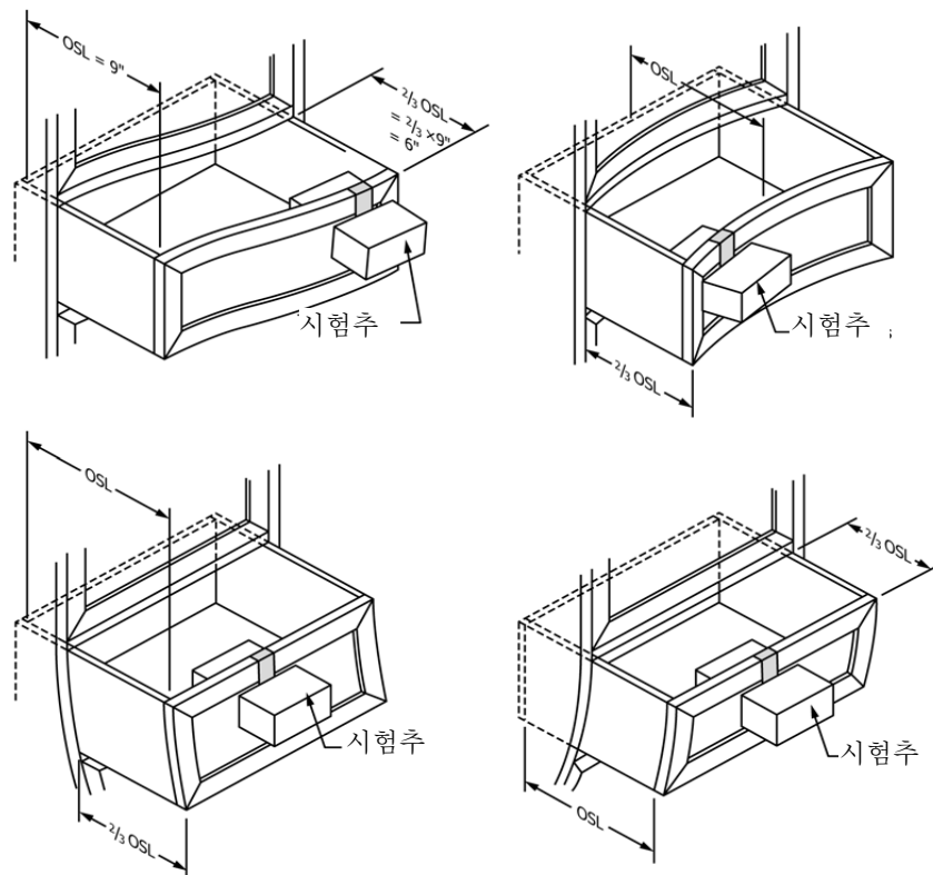
그림 19 — 서랍의 시험 하중 위치 보기
