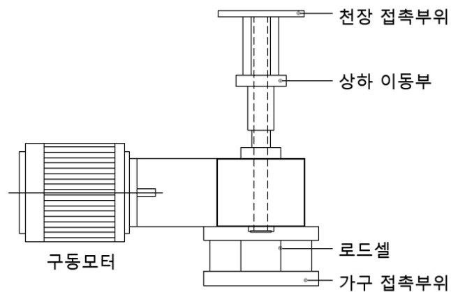
그림 A.2 — 하중을 가하는 장치의 예시
