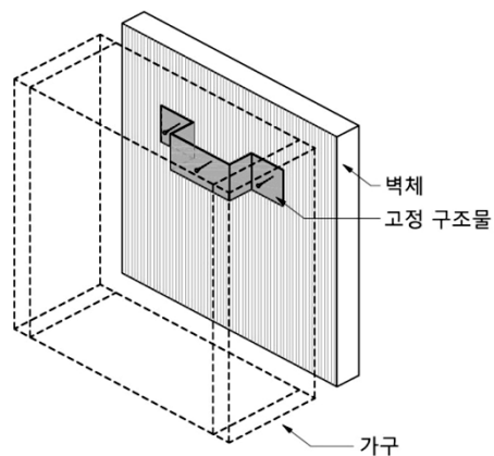
그림 9 — 전도 방지물의 적용 위치
