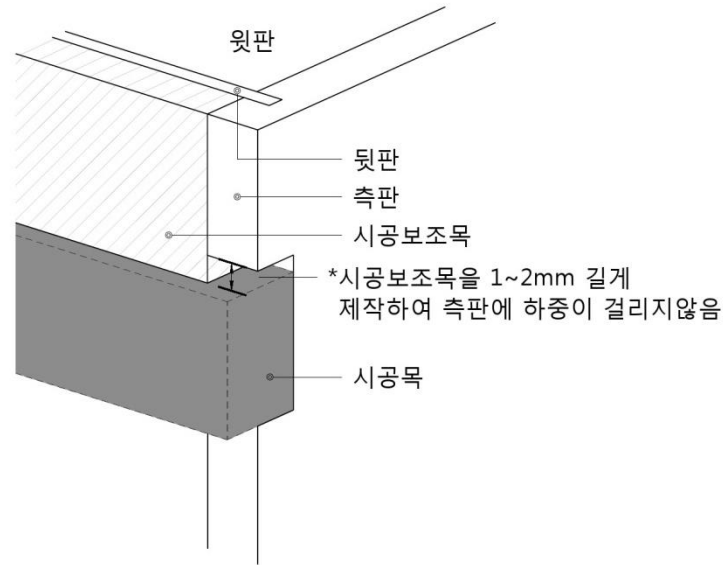
그림 D.4 — 시공보조목 길이
