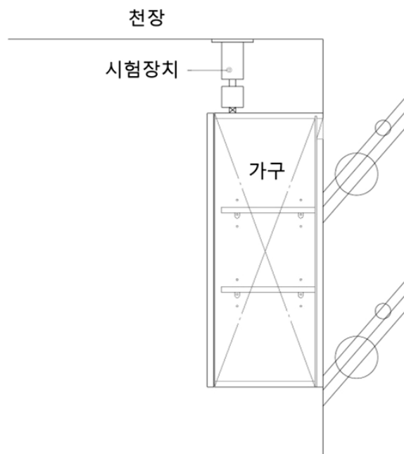
그림 13 — 추락 안정성 시험
