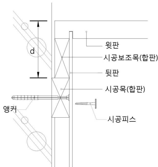
그림 D.1 — 벽장 따내기
