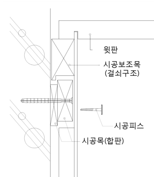
그림 D.2 — 결쇠구조
