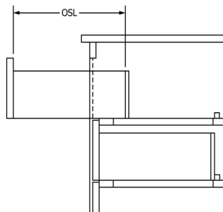
그림 18 — 작동길이
