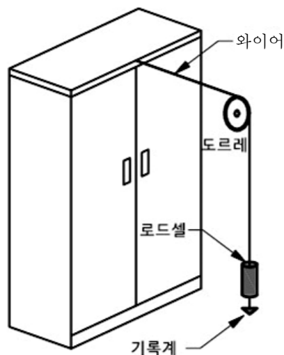
그림 B.1 — 전도 시험용 장치의 예시
