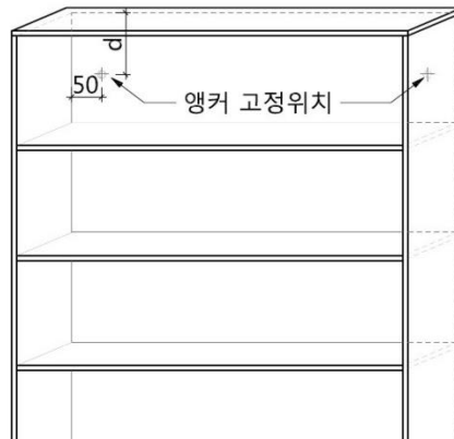
그림 7 — 앵커 고정 위치
