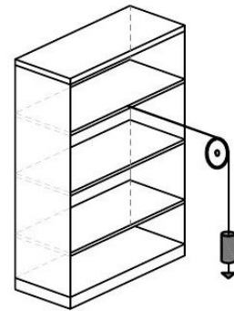
그림 16 — 선반에 하중을 가함
