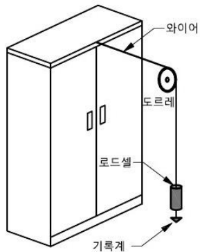
그림 14 — 몸체에 하중을 가함
