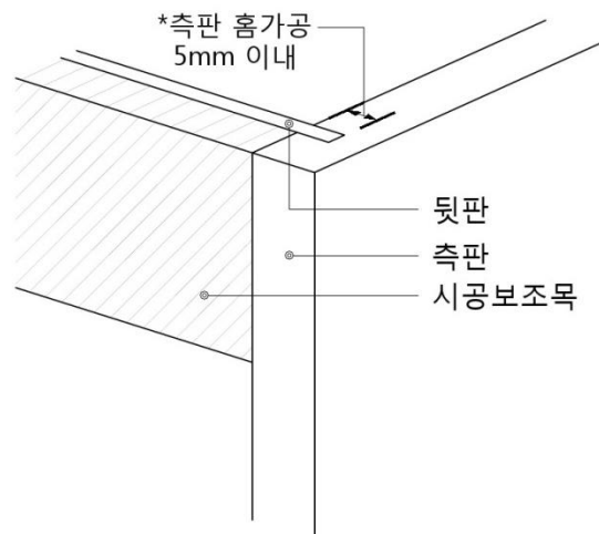
그림 D.3 — 측판 홈가공
