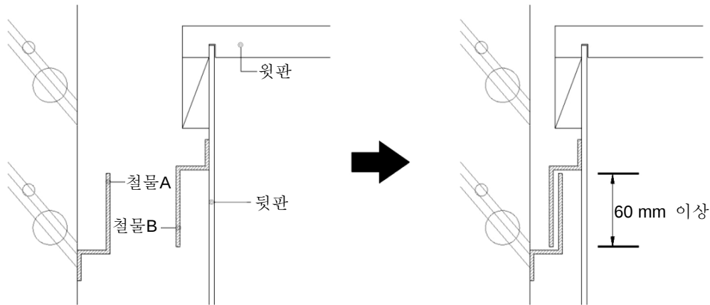
그림 2 — 행거타입 보기
