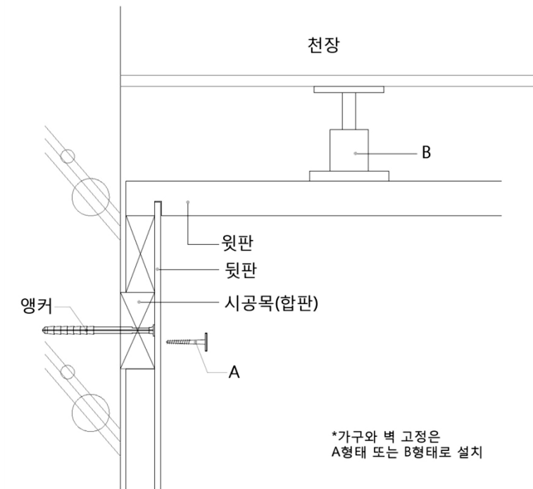
그림 C.2 — 배치식 가구의 고정 방법
