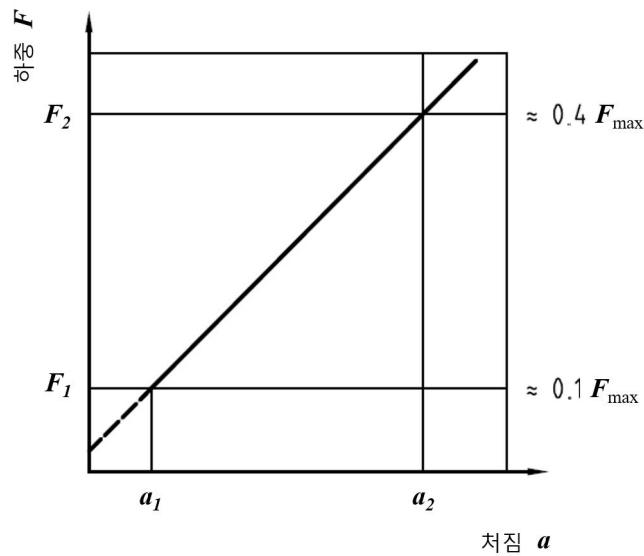
그림 6 - 탄성 변형 구간에서의 하중-처짐 곡선
