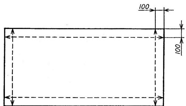
그림 5 - 너비 및 길이 측정
